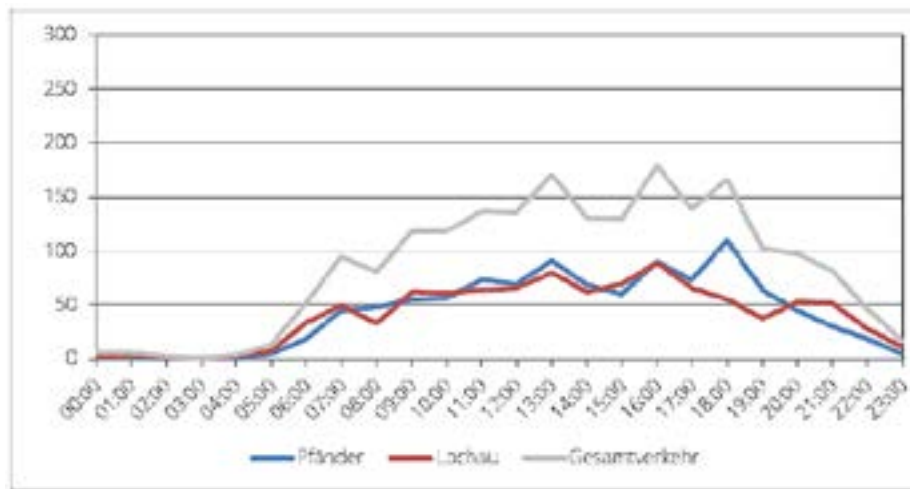
Abb. 9: Tagesganglinie am QS Jesuheim, Gesamtquerschnitt für Do, 12.06.2025
